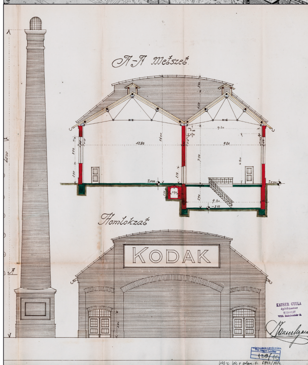
A Kodak gyár legjellegzetesebb építménye, a kazánház és a kémény tervrajza (1914) / The blueprint of the most characteristic building of the Kodak factory, that of the boiler-house and the chimney
